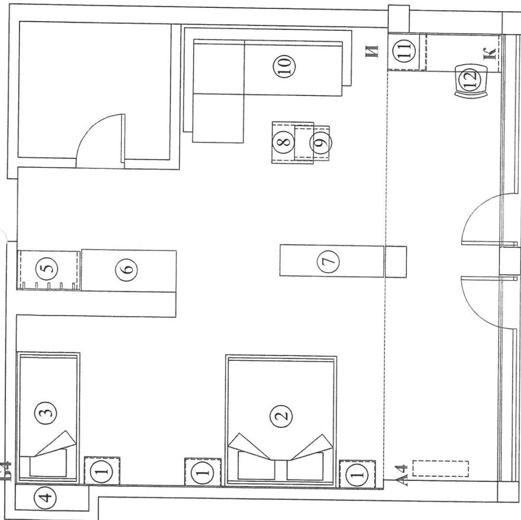
РАЗПРЕДЕЛЕНИЕ , М 1:50 апартамент 429
