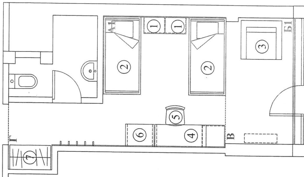
РАЗПРЕДЕЛЕНИЕ, М 1:50
