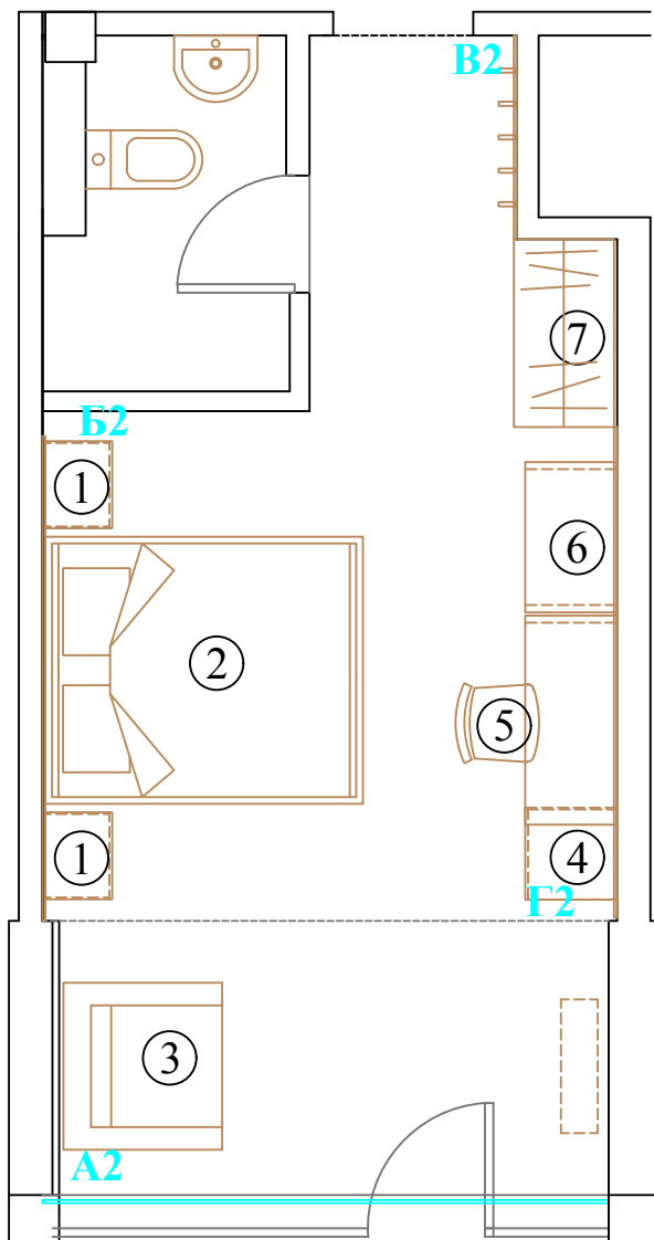
РАЗПРЕДЕЛЕНИЕ , М 1:50
