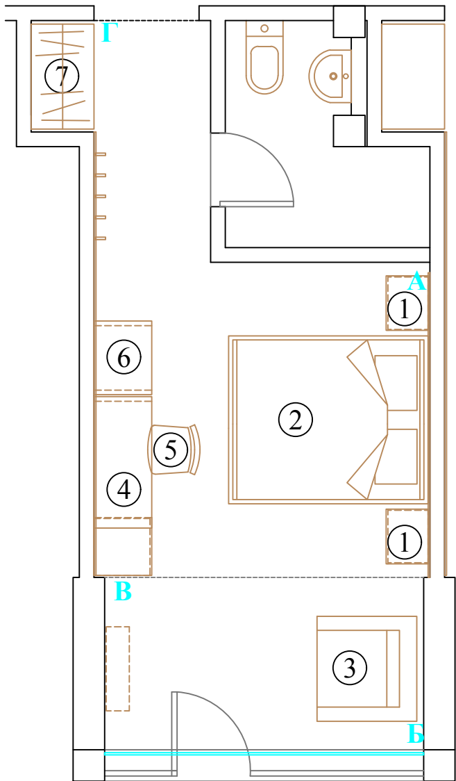
РАЗПРЕДЕЛЕНИЕ , М 1:50
