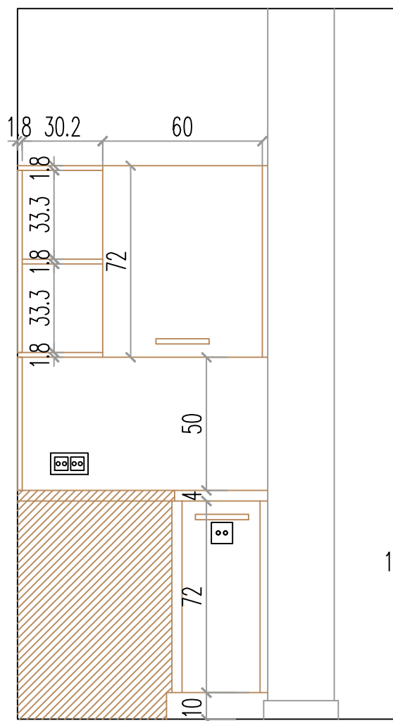
РАЗГЪВКА Ж-З
