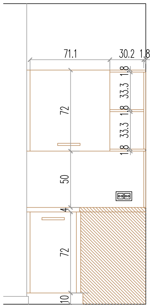
РАЗГЪВКА Д-Е
