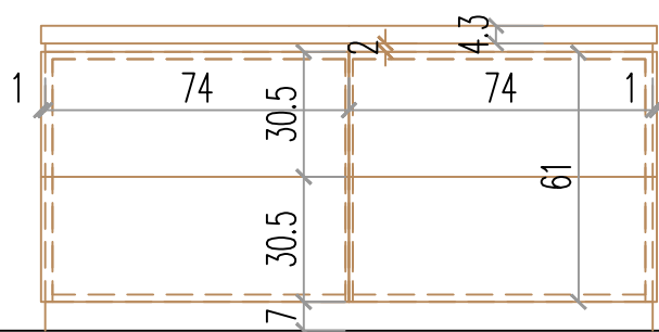
скрин 150/52/74 Н
