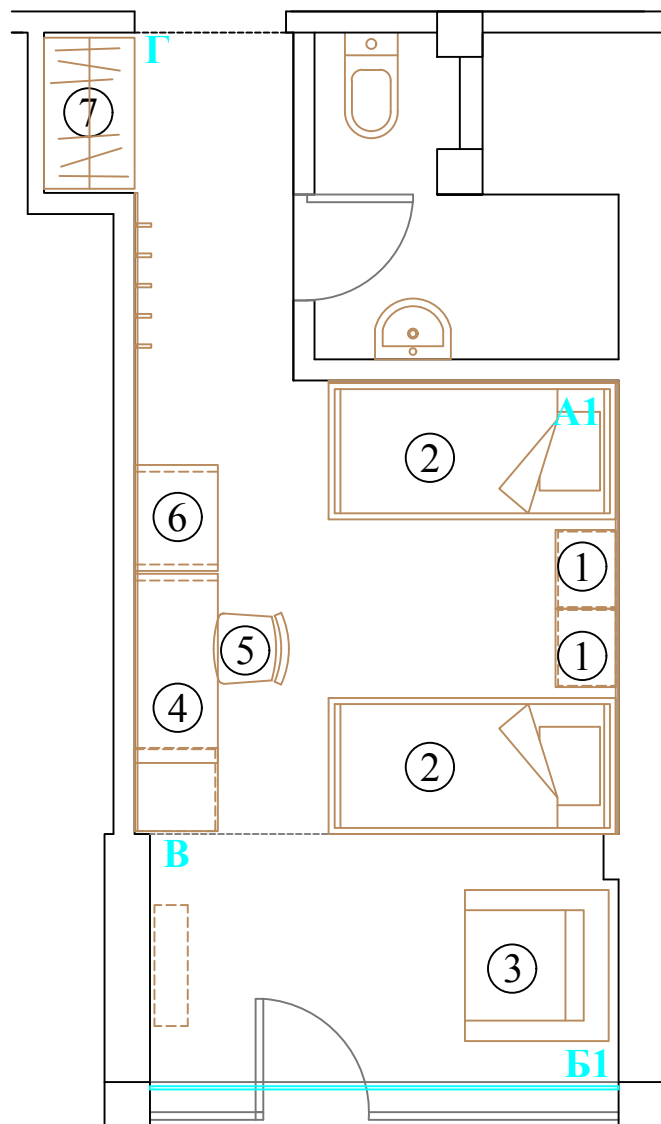
РАЗПРЕДЕЛЕНИЕ, М 1:50
